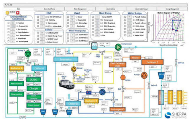
Banc numérique
